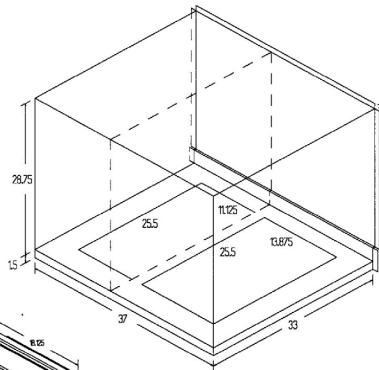
PCP101-103 PLENUM
