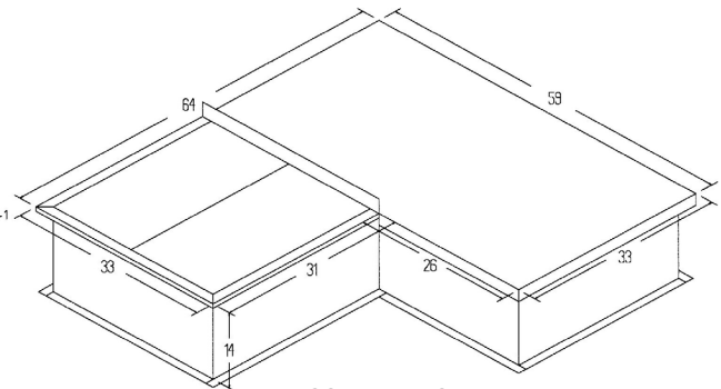
PCCP101-103 CURB
